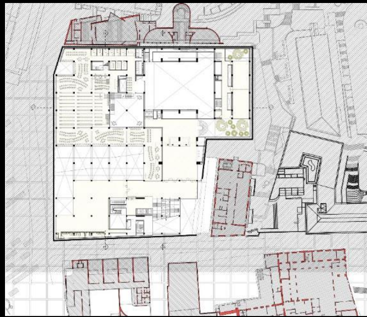
PLANTA NIVEL 01
