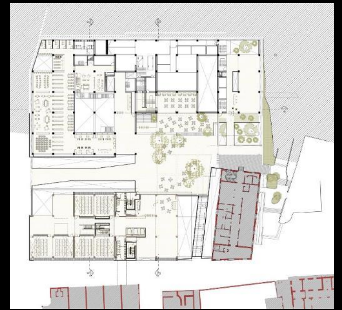
PLANTA NIVEL 02
